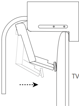
TV 상단에 설치하기
