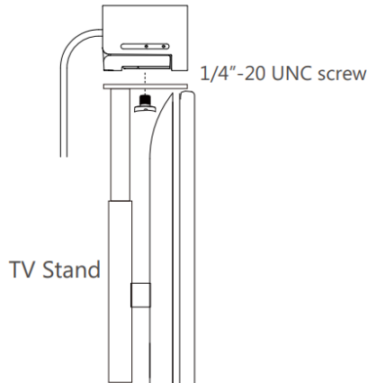
TV 거치대 또는 삼각대 상단에 설치하기
